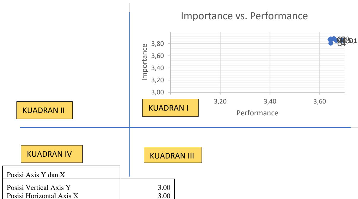
Gambar 10: Grafik Kuadran Tingkat Kepentingan (Importance) vs Kinerja Pelayanan (Performance)
